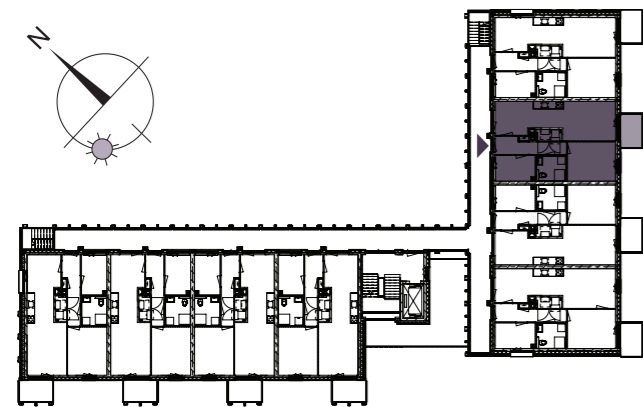
Appartement Bnr. 147 | 2 e verdieping
